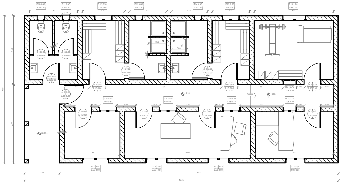
— ΚΑΤΟΨΗ —
