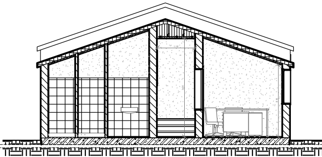
— ΤΟΜΗ Α-Α' —
