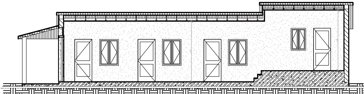
— ΤΟΜΗ Γ-Γ' —
