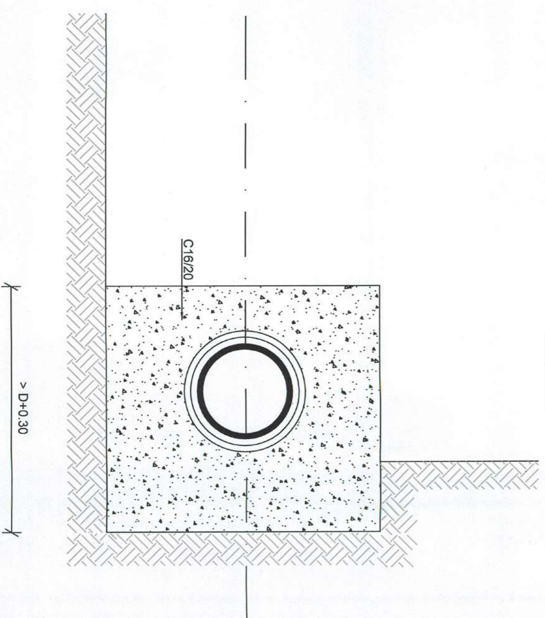
ΤΟΜΗ Α-Α
