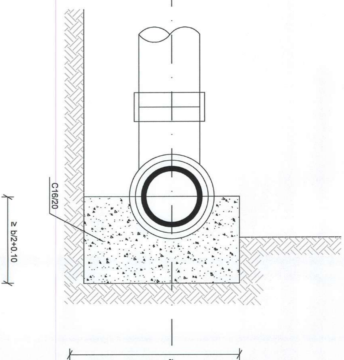
ΤΟΜΗ Α-Α
